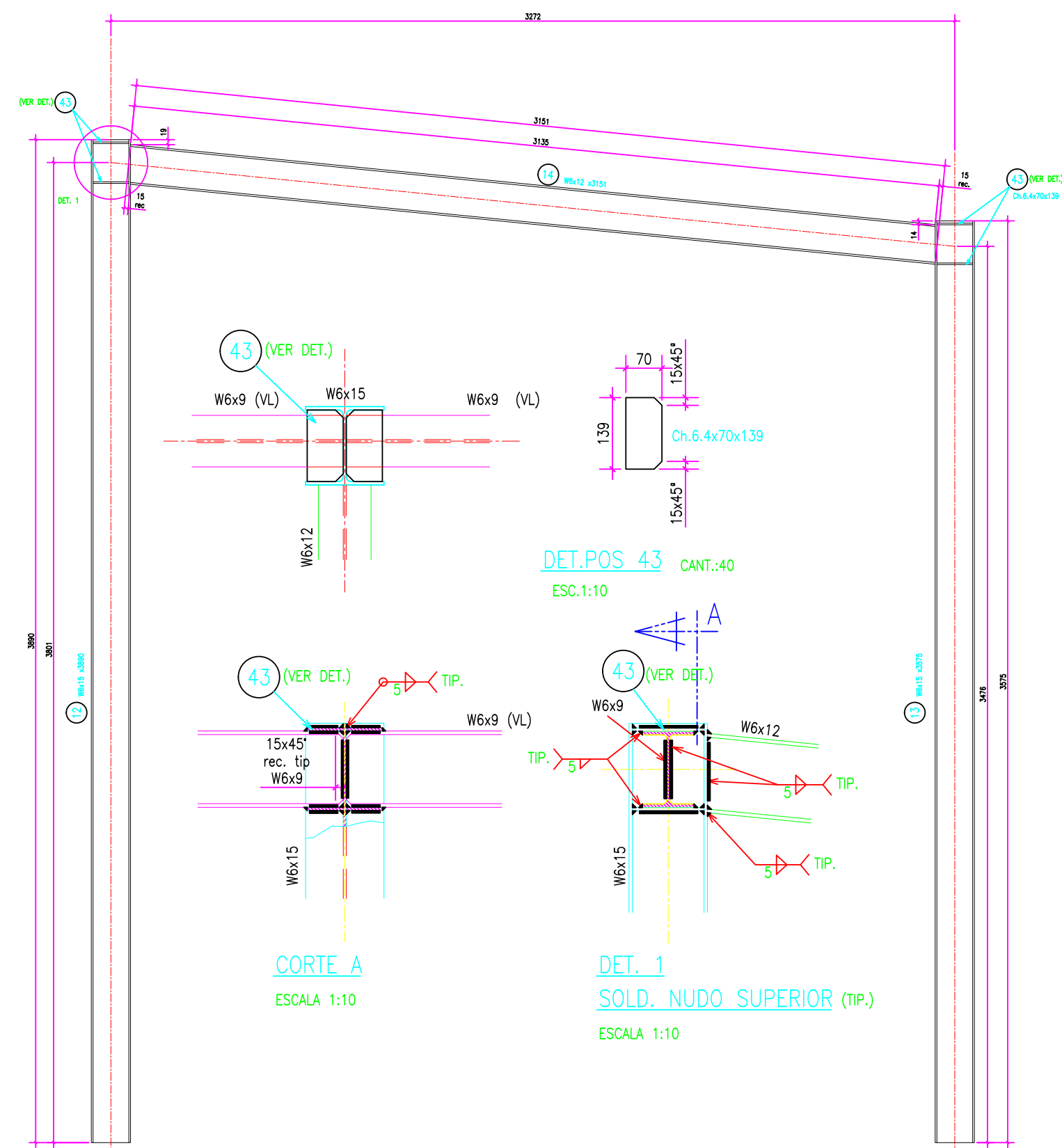
DET. POS. 43 ESC. 1:10
