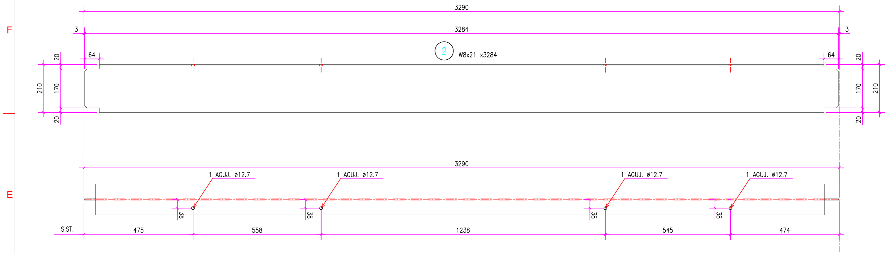
CORREAS LATERALES ESCALA 1:10
