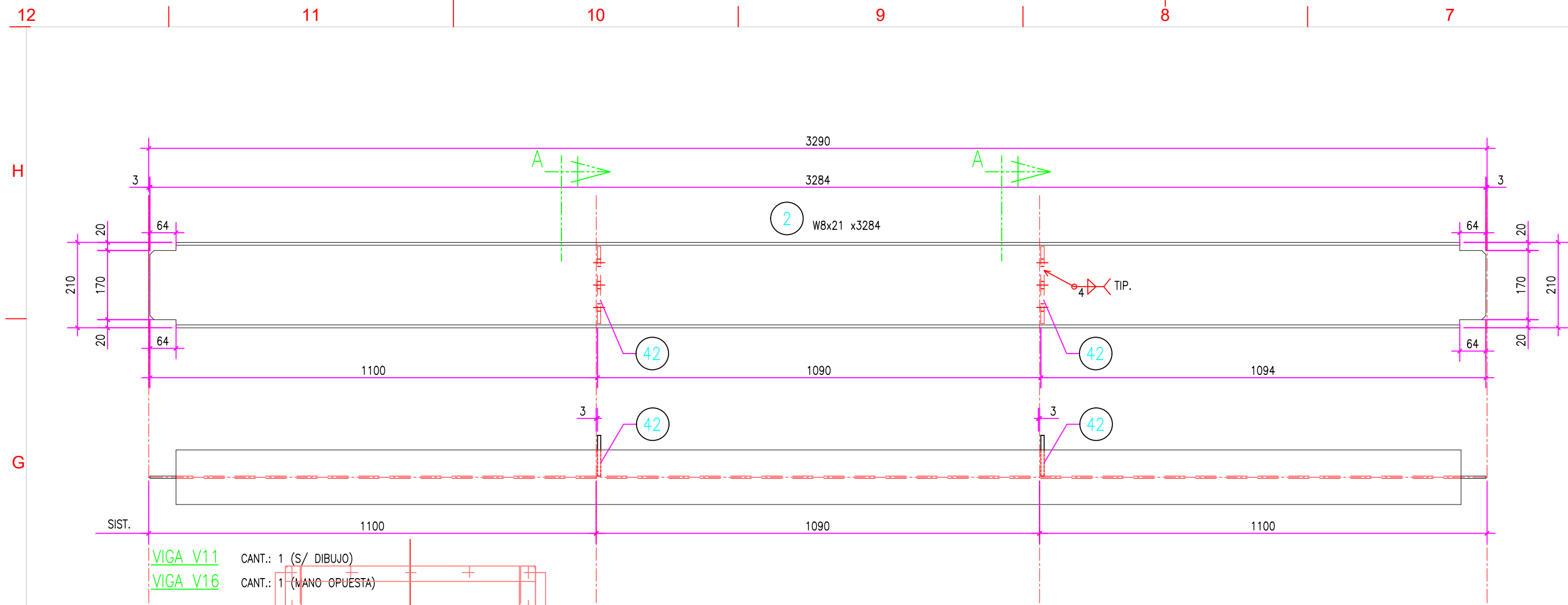
CORREAS FRONTS ESCALA 1:10
