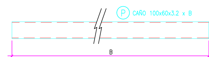
CORREAS TERCHO ESCALA 1:10
