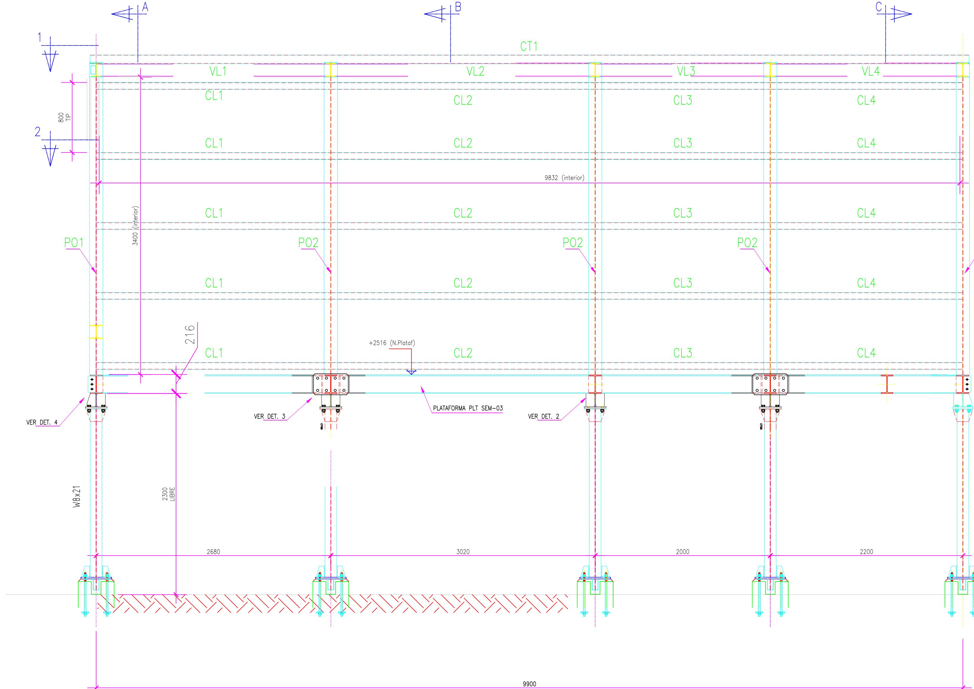
VISTA LATERAL SEM-03 ESCALA 1:25
