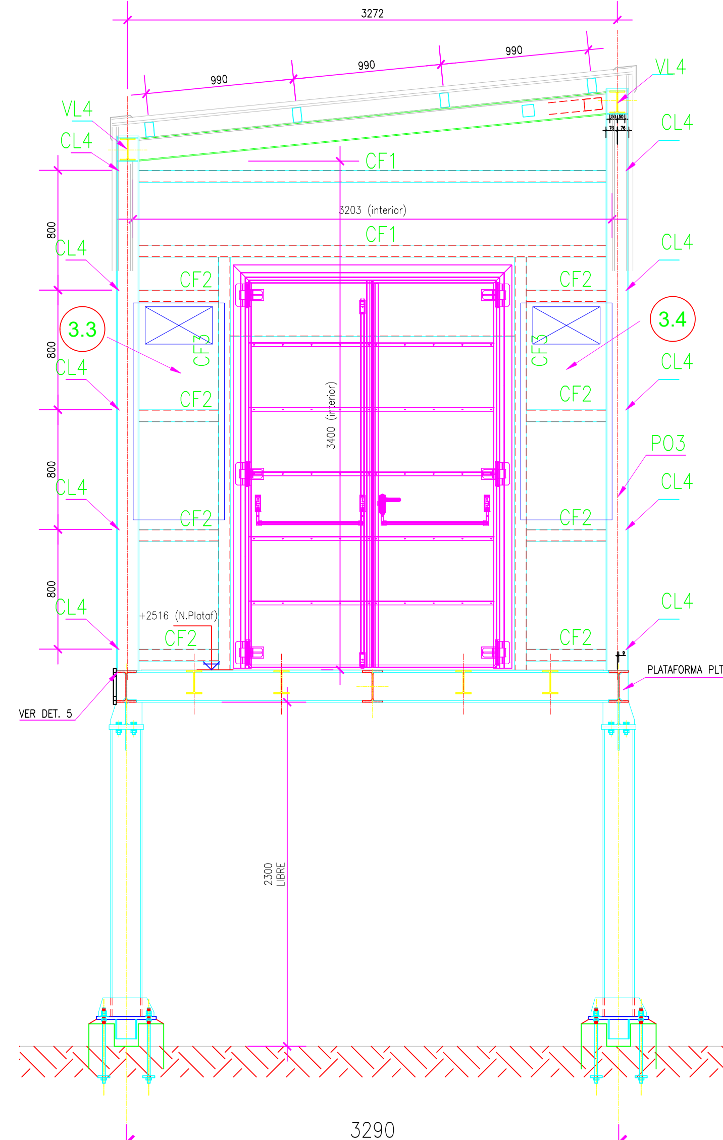
CORTE C-C SEM-03 ESCALA 1:25
