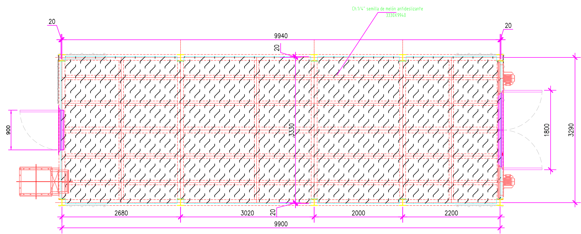
PLANTA CHAPA DE PISO PLATAFORMA PLT SEM-03 ESCALA 1:50
