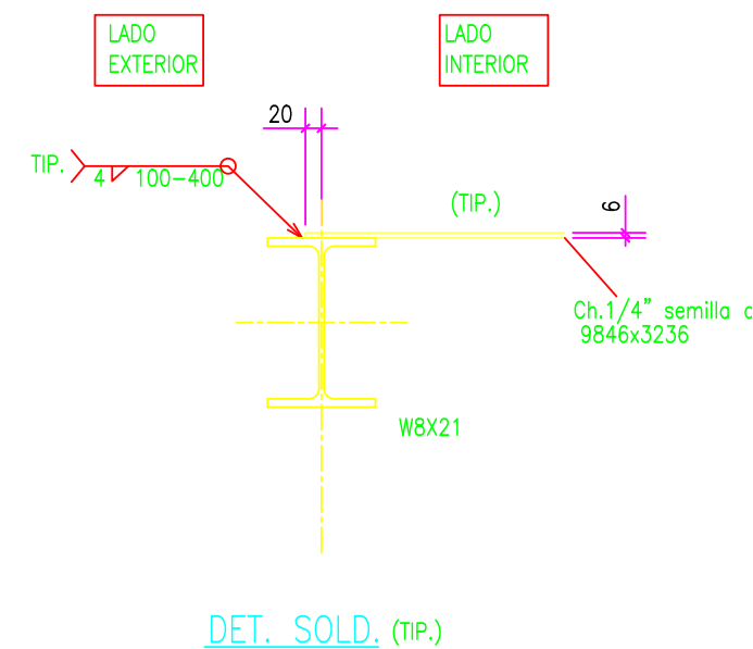
DET. SOLD. (TP.)
