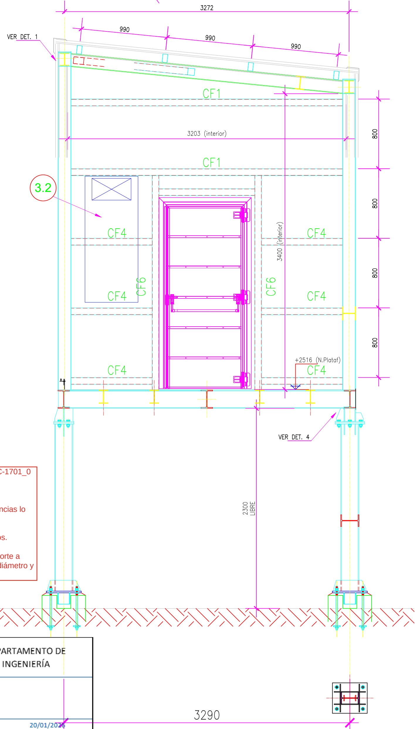
CORTE A-A SEM-03 ESCALA 1:25
