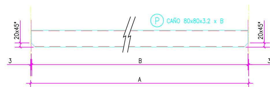
CORREAS FRONTS ESCALA 1:10
