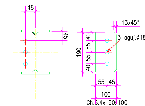
DET. POS. 42 ESC. 1:10
