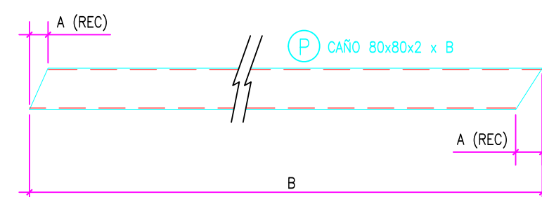
CORREAS TERCHO ESCALA 1:10
